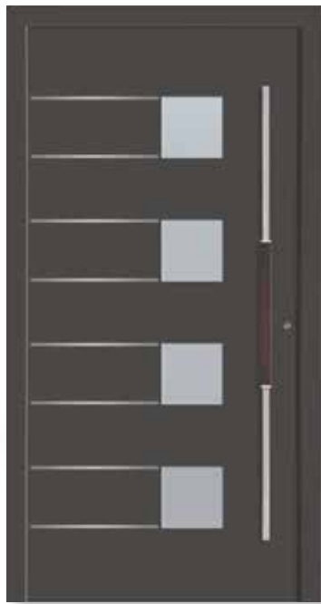
M-230 Ansicht A / DIN rechts [J] Applikationen in Edelstahloptik außen und Rahmen in Edelstahloptik innen ■ Aufsatzfüllung ■ Farbe Eisenglimmer ähnl. DB 703 Feinstruktur ■ Isolierglas Satinato weiß | GG 2 ■ Griff ZAE 164, 1600 mm | PG 16 (Holzelement variabel einstellbar)
