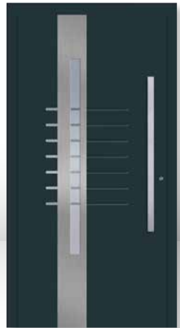
M-237 Ansicht A / DIN rechts K Nuten und Applikation in Edelstahloptik außen
